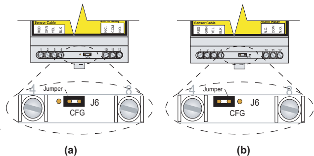
Abbildung 8. CFG Stecker Position zur Konfiguration (a) und normalen Betrieb (b)
