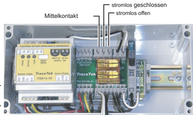
Abbildung 5. Relaisanschluss
