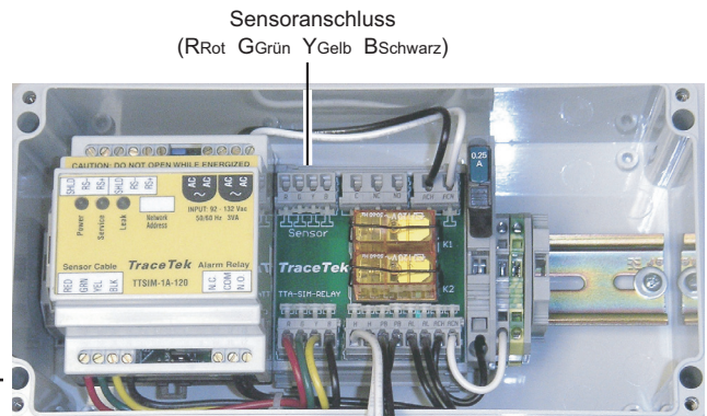
Abbildung 4. Anschluss der Sensorkabel
