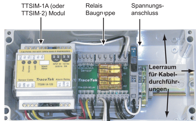
Abbildung 2. Leerraum für Kabeldurchführung
