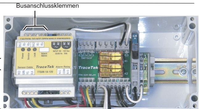
Abbildung 6. Busanschluss
