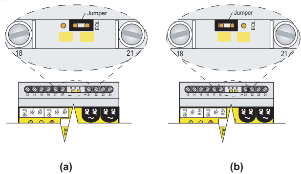
Abbildung 7. Position des Endjumpers EOL für den letzten TTSIM (a) und alle anderen TTSIM (b)
