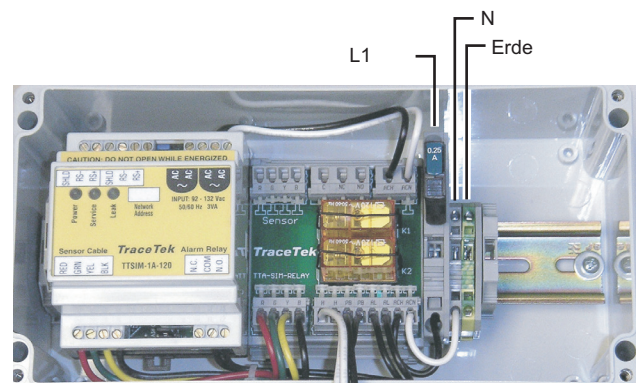
Abbildung 3. Anschluss Spannungsversorgung
