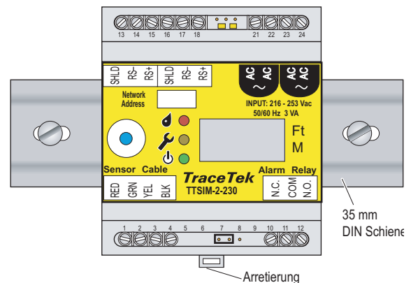
Abbildung 1. Montage auf DIN-Schiene
