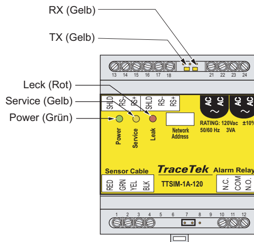
Abbildung 9. TTSIM-2 LED Position
