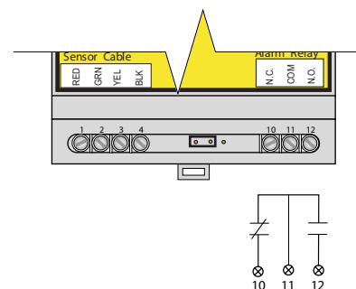
Abbildung 4. Alarmrelaiskontakt (Darstellung spannungslos)
