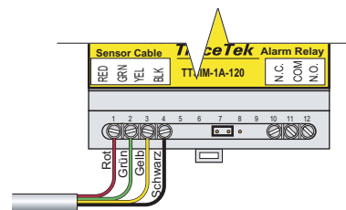
Abbildung 6. Anschluss der Sensorkabel
