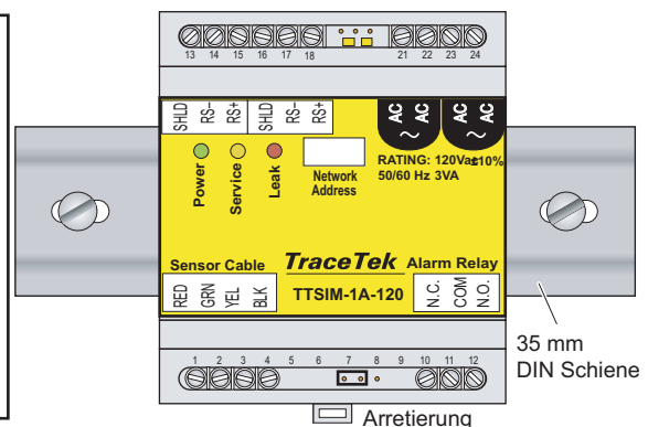
Bild 1 Montage auf DIN-Schiene
