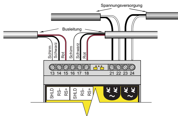
Bild 3 Spannungsversorgung und Busanschluss
