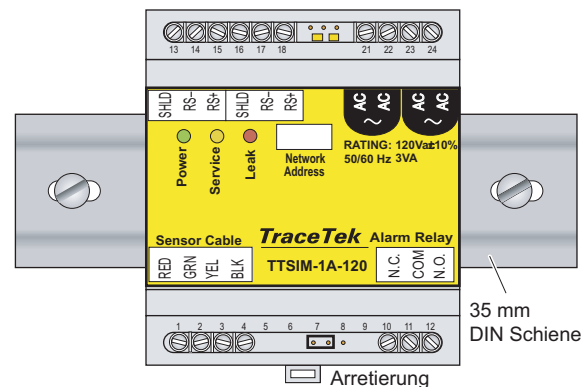
Bild 7b Konfigurationsjumper in Betriebsposition
